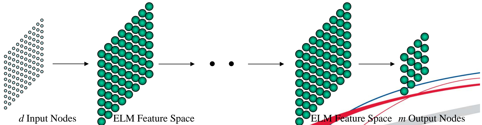
ELM
