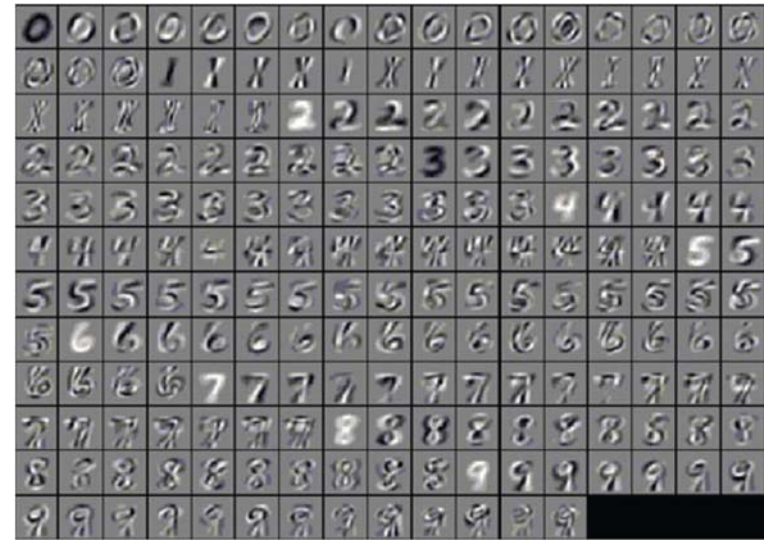
(b) SVD
