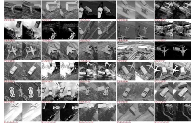
NORB Dataset
