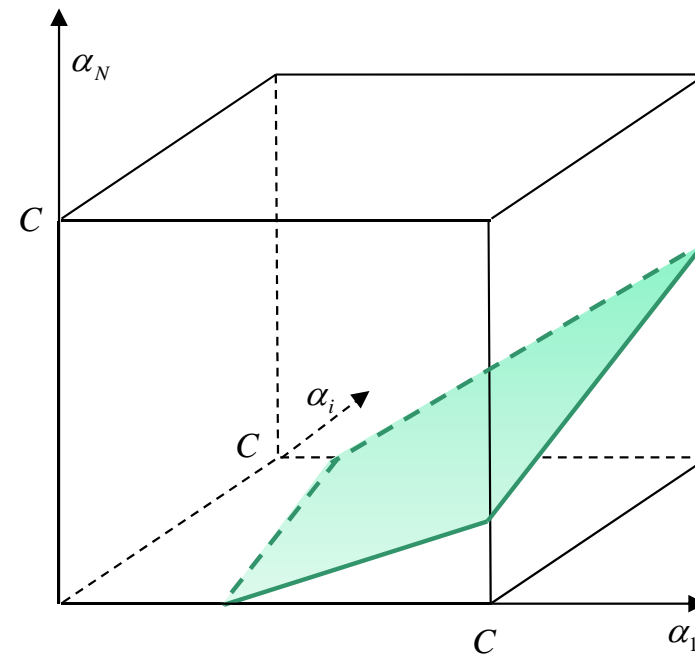
SVM
